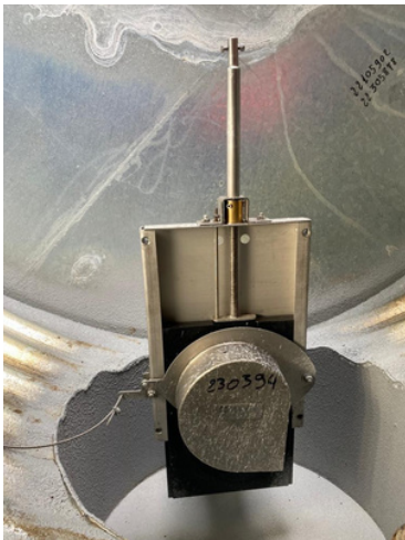
Vanne de confinement avec régulation de débit (ouvrage mixte)
